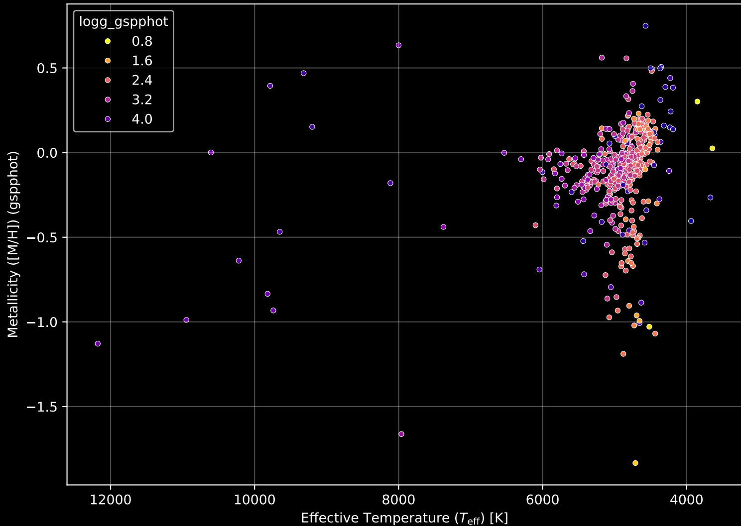
APOGEE DR17 Field: [090-08] Stellar Population Parameters (n= 493)
